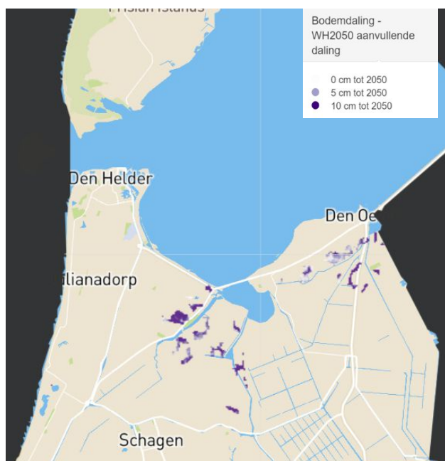
Figuur 2-9 Verwachte aanvullende bodemdaling bij het klimaat van 2050. Bron: hhnk.klimaatatlas.net
