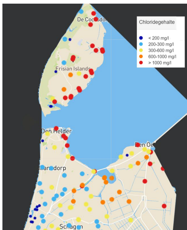
Figuur 2-10 Gemeten chloride-gehalten (een maat voor de verzilting) in de zomers van 2013 en 2015. Bron: hhnk.klimaatatlas.net
