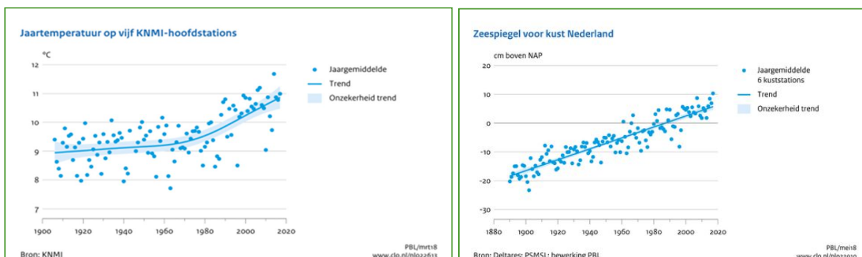
Figuur 2-1 Trend in jaargemiddelde neerslaghoeveelheid in de afgelopen eeuw (links) en neerslagtekorten in de zomers van 1976, 2018 en 2020 (rechts)
