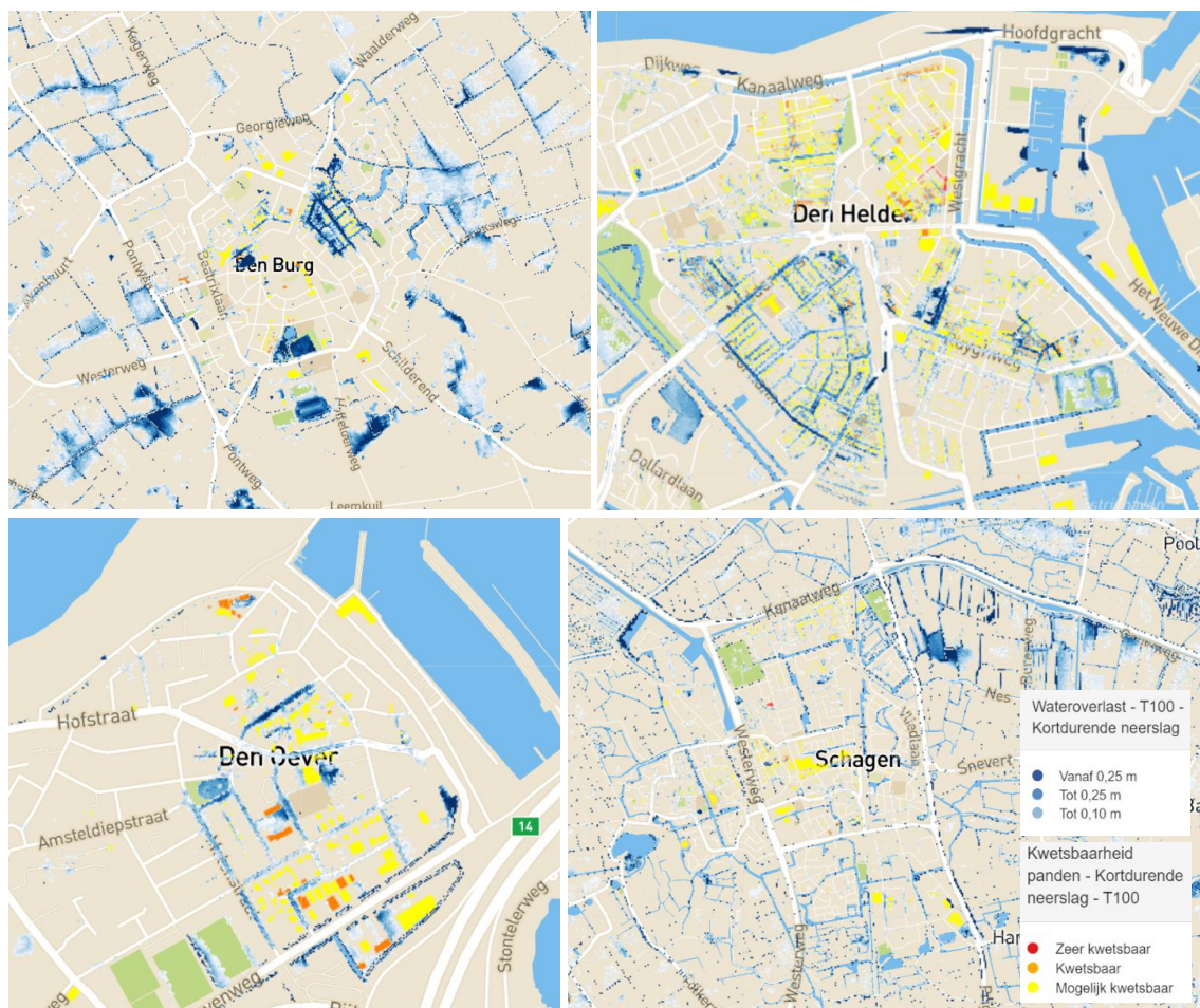
Figuur 2-4 Risico's op wateroverlast in de kernen: Den Burg en Den Helder (boven) en Den Oever en Schagen (onder) De waterdiepten volgen uit modelberekeningen van een set korte en langdurige buien: van 81 mm in 2 uur tot 135 mm in 2 dagen, bij verschillende grondwaterstanden. De kwetsbaarheid panden geldt voor een bui van 100 millimeter in 2 uur. Bron: hhnk.klimaatatlas.net
