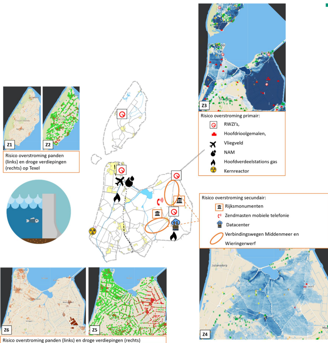
Figuur 4-4 De opgaven bij overstromingen vanuit primaire en secundaire keringen
