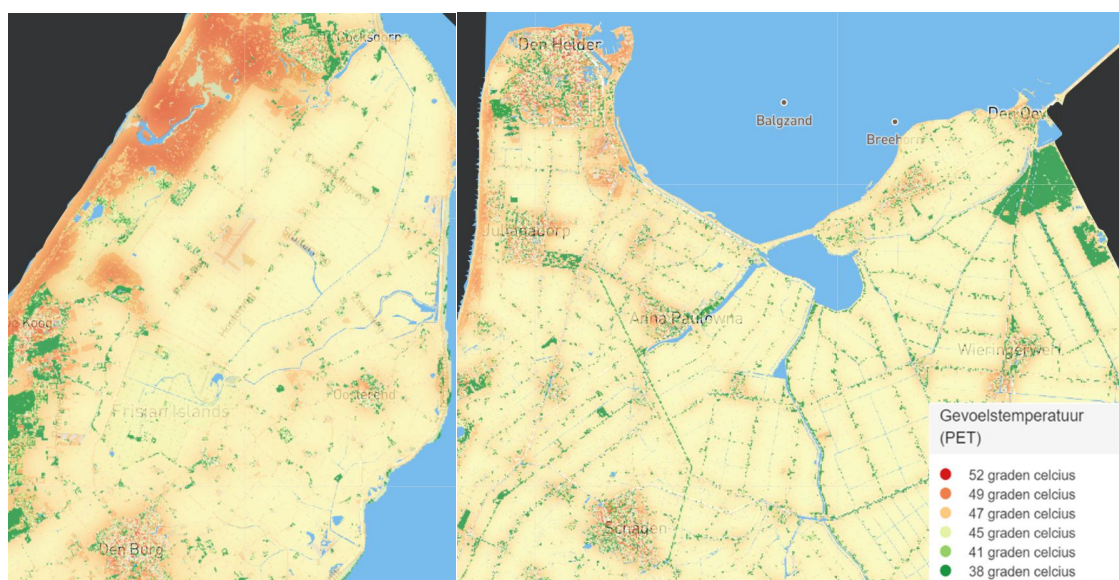
Figuur 2-8 Gevoelstemperatuur tijdens een zeer hete dag (1 juli 2015) in de Noordkop. Bron: hhnk.klimaatatlas.net
