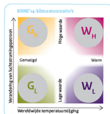
Figuur 2-3 Visualisatie van de vier KNMI-klimaatscenario's
