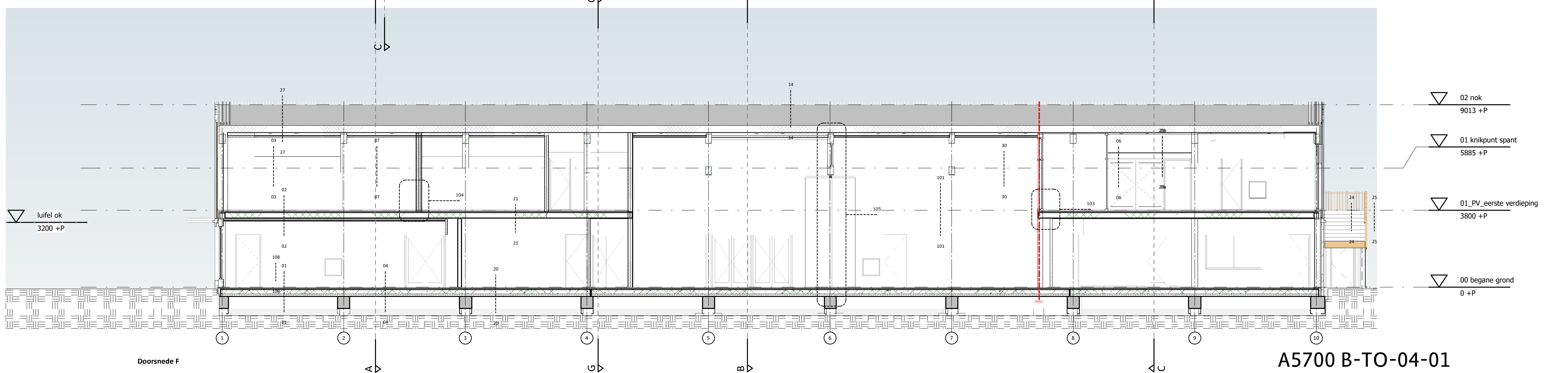
Doorsnede E
