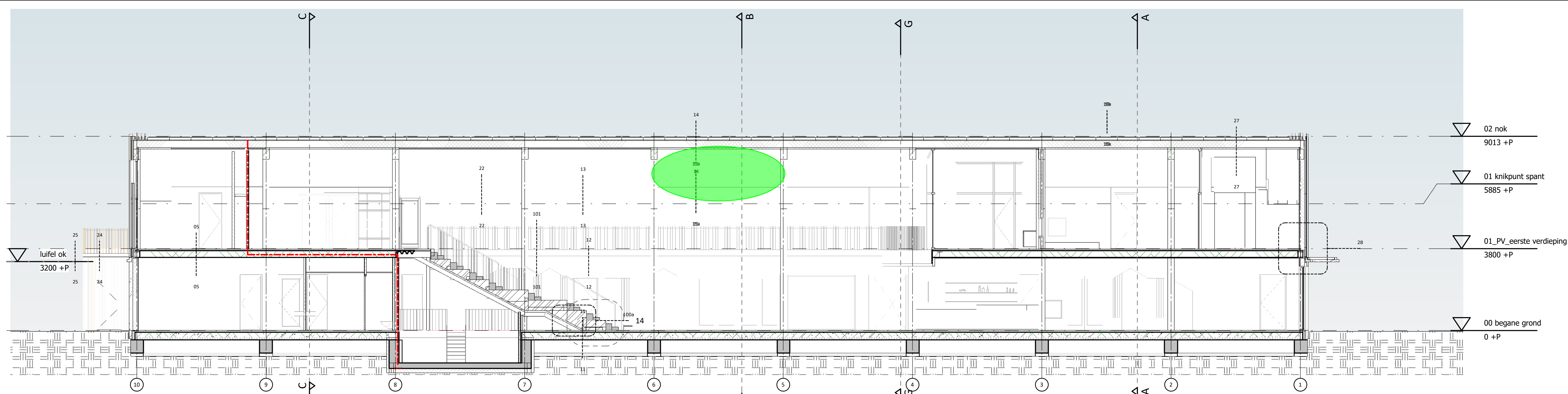
Doorsnede D
